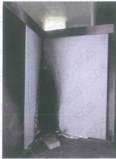
After Test (EN 13823)
